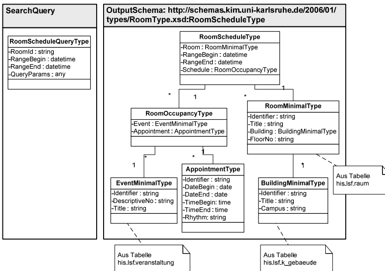
Abbildung 4: Aufruf- und Rückgabeparameter der Raumbelegungssuche
