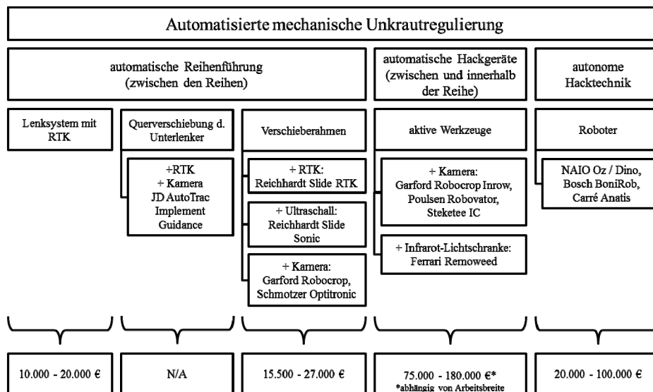
Abb. 1: Systematisierung von verfügbaren Technologien sowie Prototypen zur automatisierten mechanischen Unkrautregulierung
