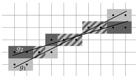
Abbildung 6: Beispiel zweier digitaler Strecken, deren Schnitt (schraffiert) nicht zusammenhängt.
