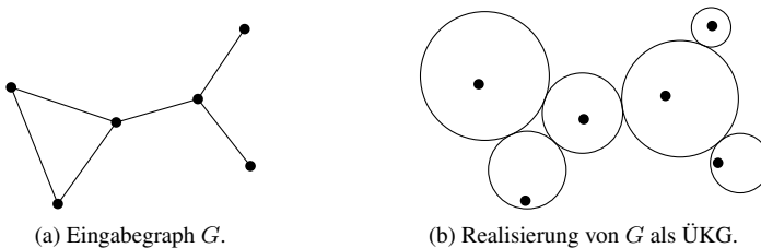
Abbildung 5: Realisierung eines Graphen als Überdeckungskontaktgraph.
