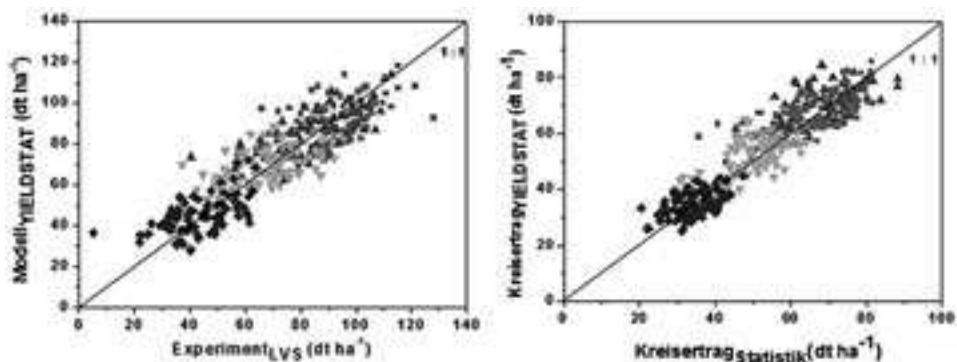
Abbildung 1: Ertragsvergleich zwischen Modell YIELDSTAT und Feldversuch (links) bzw. Kreisstatistik (rechts) für Winterweizen (■), Wintergerste (▲), Sommergerste (▼) und Winterraps (◆) für den Zeitraum 1995-2010
