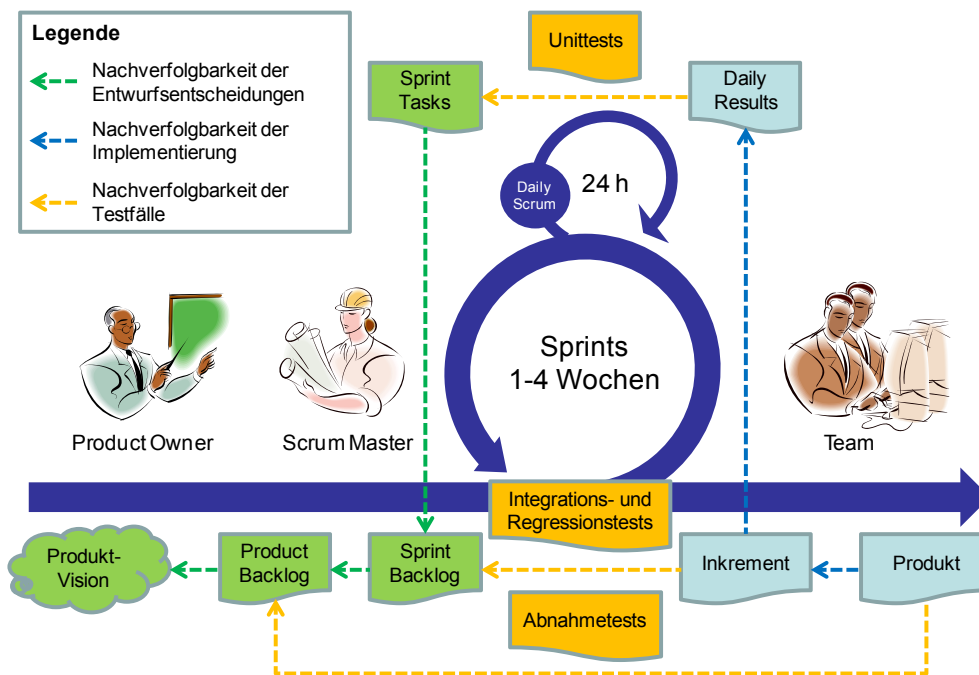
Abbildung 1. Traceability Architekturartefakte im erweiterten Scrum
