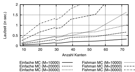
Abbildung 3: Vergleich der Laufzeiten bei Monte Carlo Simulation
