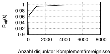
Abbildung 1: Entwicklung von R_{All} in Abhängigkeit von der Anzahl der betrachteten Komplementärereignisse s \in \underline{T}
