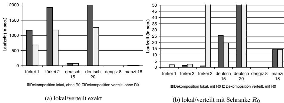
Abbildung 2: Vergleich Laufzeiten Dekompositionsansatz lokal/verteilt
