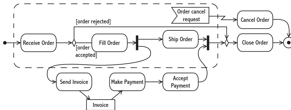
Abbildung 3: Beispiel für eine InterruptibleActivityRegion im Standard.
